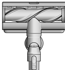
Spazzola digital Motorbar™ con pettine anti-groviglio La tecnologia Dyson DLS™ monitora la resistenza della spazzola e adatta la potenza di aspirazione a diversi tipi di superfici. I denti in policarbonato impediscono la formazione di grovigli attorno alle setole.
